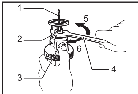
► 1. Embout 2. Ecou à collet 3. Verrouillage de l'arbre 4. Clé 5. Desserrer 6. Serrer
