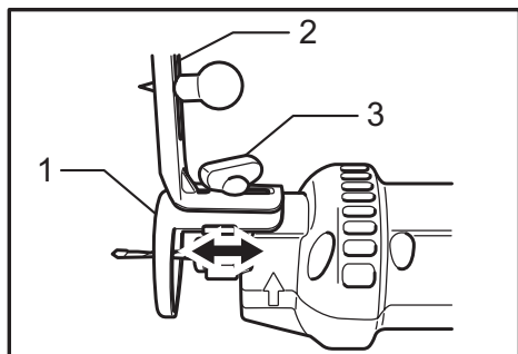
► 1. Sabot 2. Guide circulaire 3. Vis à oreilles
