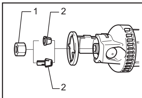
► 1. Ecou à collet 2. Cône de la bague de mandrin
