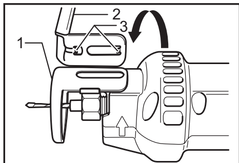
► 1. Sabot 2. Guide circulaire 3. Parties saillantes
